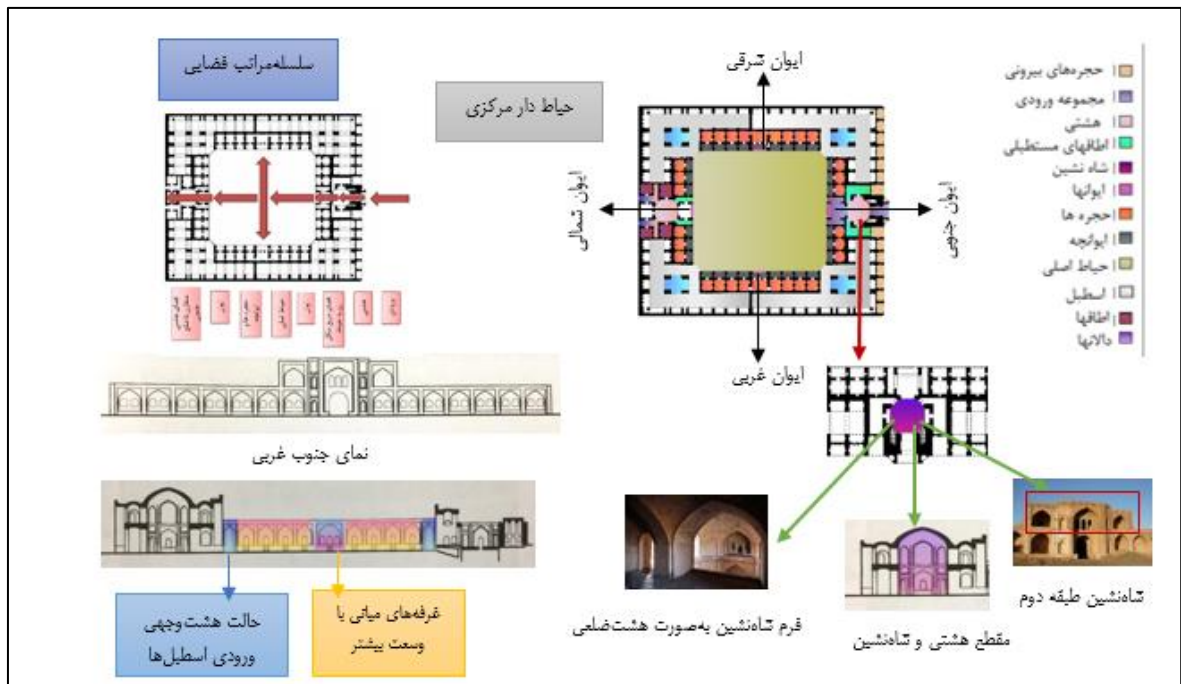
شکل ۱۷: نقشه‌ها و تصویر کاروانسرای مهر (مأخذ: نگارندگان)
