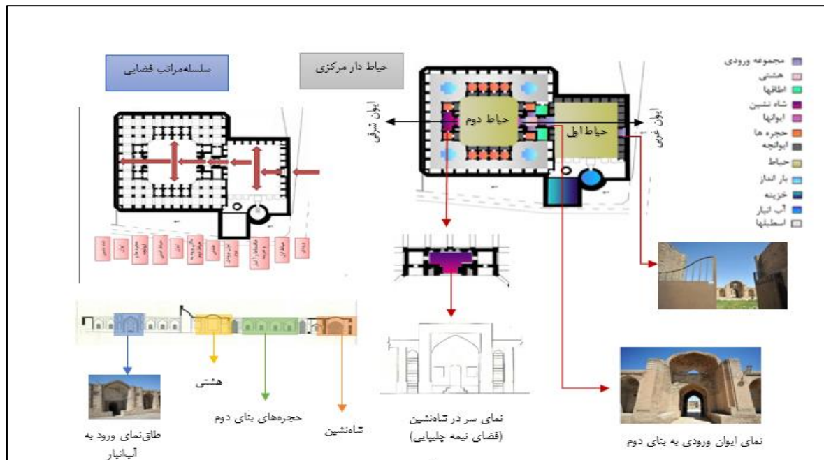
شکل ۱۱: نقشه‌ها و تصاویر کاروانسرای طرق (مأخذ: نگارندگان)
